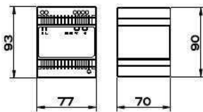
Centralina+alimentatore LED
